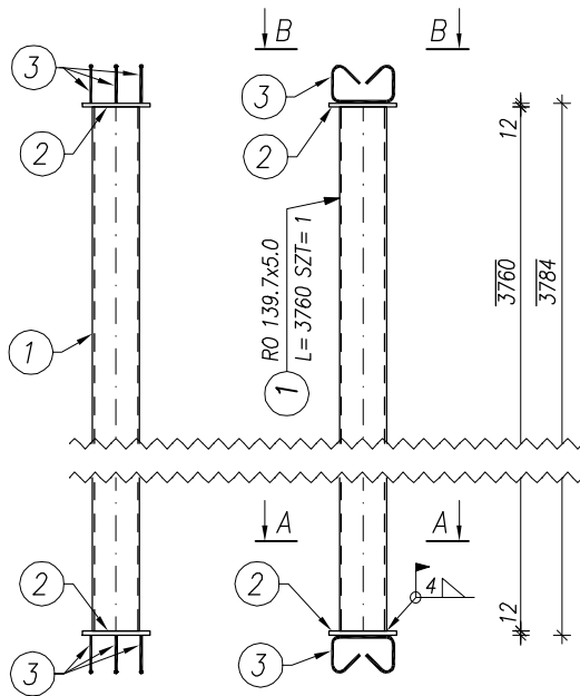
S-01 słup (szt. 2) skala 1:25
